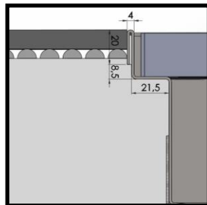
Klinker utan tätskikt (-K3)
