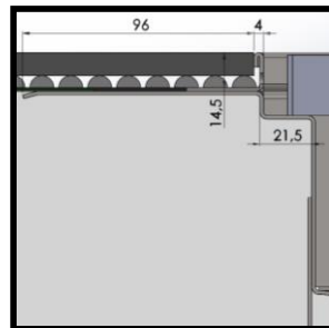
Klinker med rollat tätskikt (-K4)
