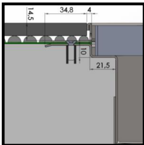
Klinker med tätskikt (-K5)
